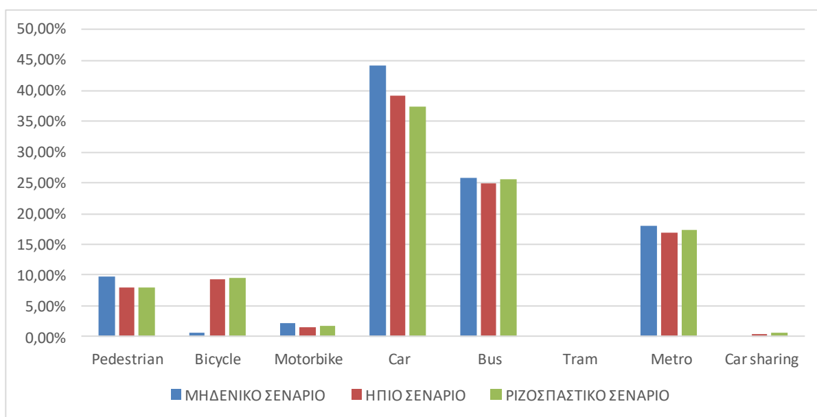
Γράφημα 3.3.2-1: Modal Split ανά σενάριο σε ορίζοντα 5ετίας
