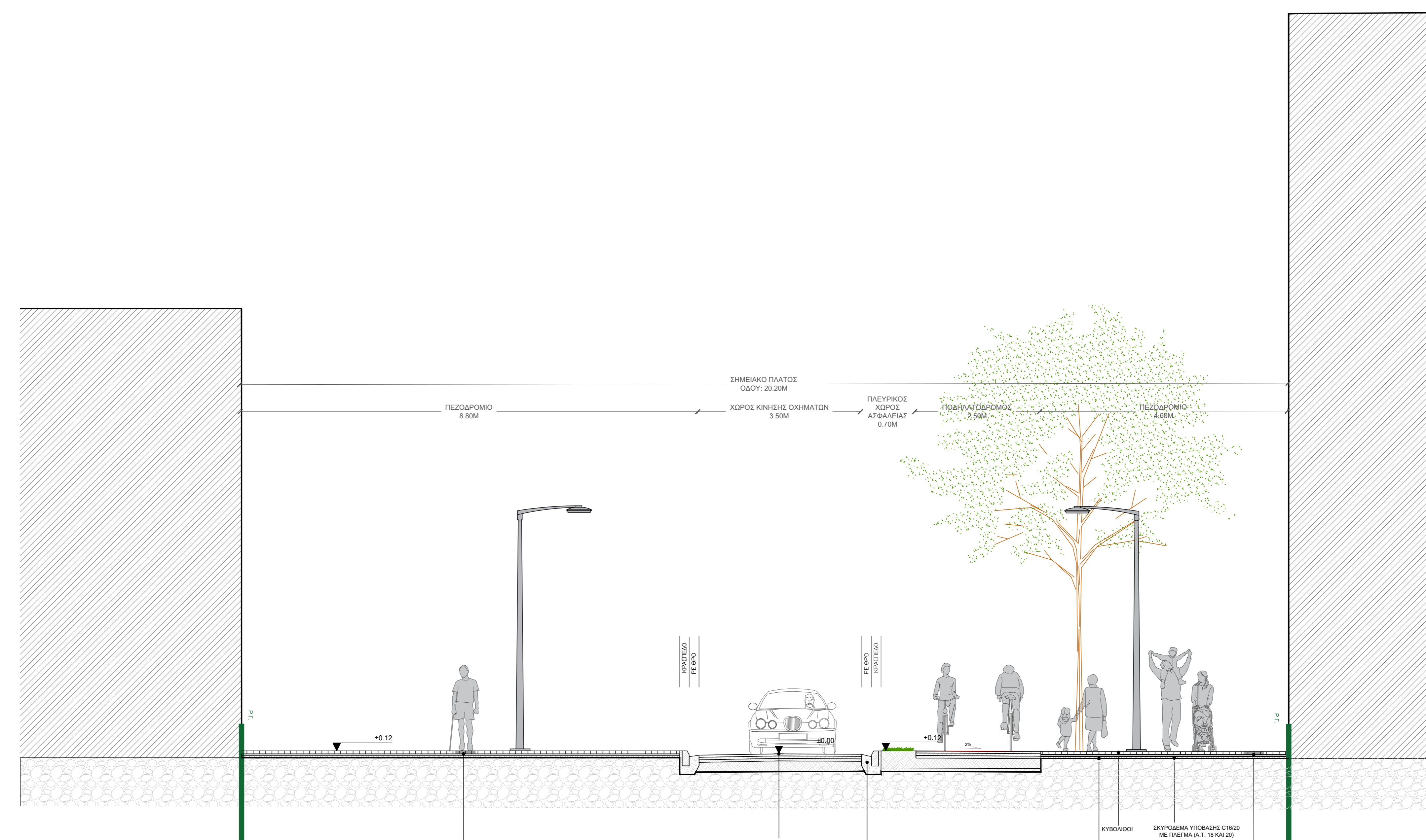
ΔΙΑΤΟΜΗ 1
