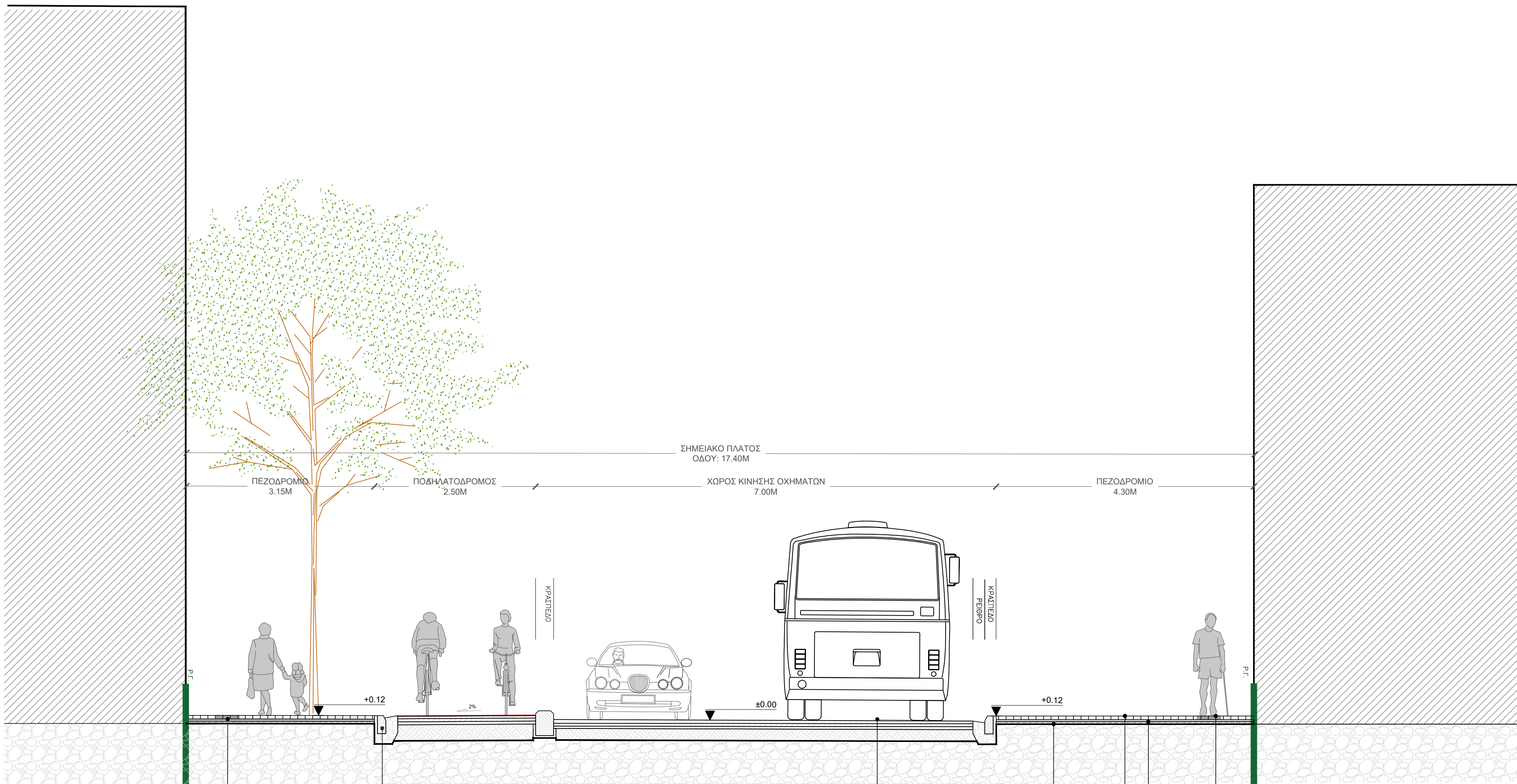
ΔΙΑΤΟΜΗ 2
