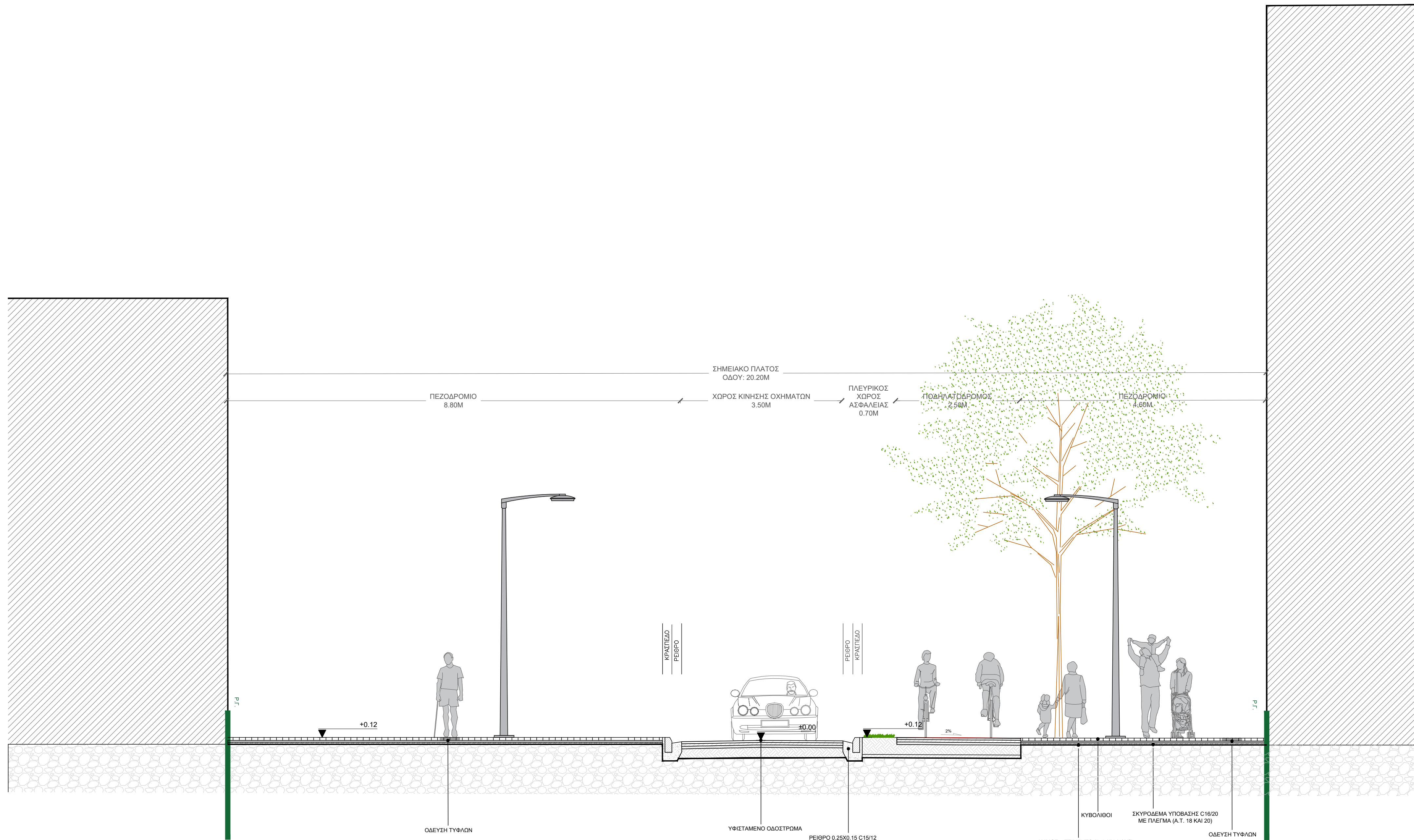
ΔΙΑΤΟΜΗ 1
